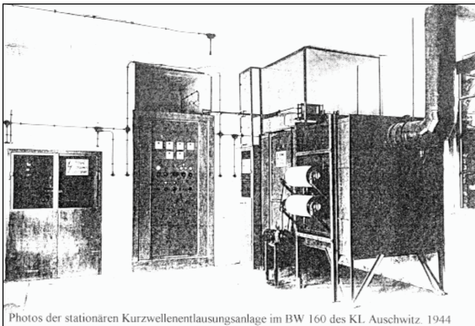
Photos der stationären Kurzwellenentlausungsanlage im BW 160 des KL Auschwitz. 1944
